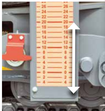
Cilindros niveladores en posición de transporte/en el último valor ajustado.
