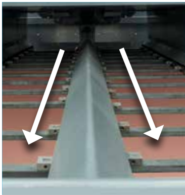
Inversión de la marcha de las cintas transportadoras de corta duración.
