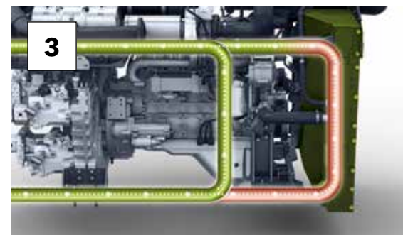
Kontrollü hidrolik yağ sıcaklığı devresi
