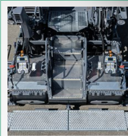
La pasarela y el acceso central bien diseñado de la solera permiten un acceso seguro y cómodo a la plataforma del operador.
