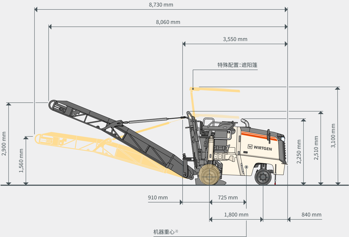
W 55 HR (i) 侧视图 / 俯视图
