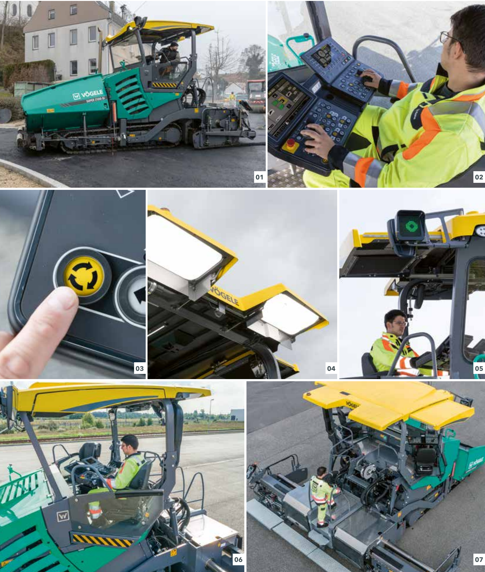
01 Diseño de producto innovador y funcional 02 ErgoPlus 5 con gran cantidad de funciones de confort y automáticas 03 AutoSet Plus para un desplazamiento más cómodo en la obra 04 Paquete de Luces Plus para la óptima iluminación de la zona de trabajo de la regla
