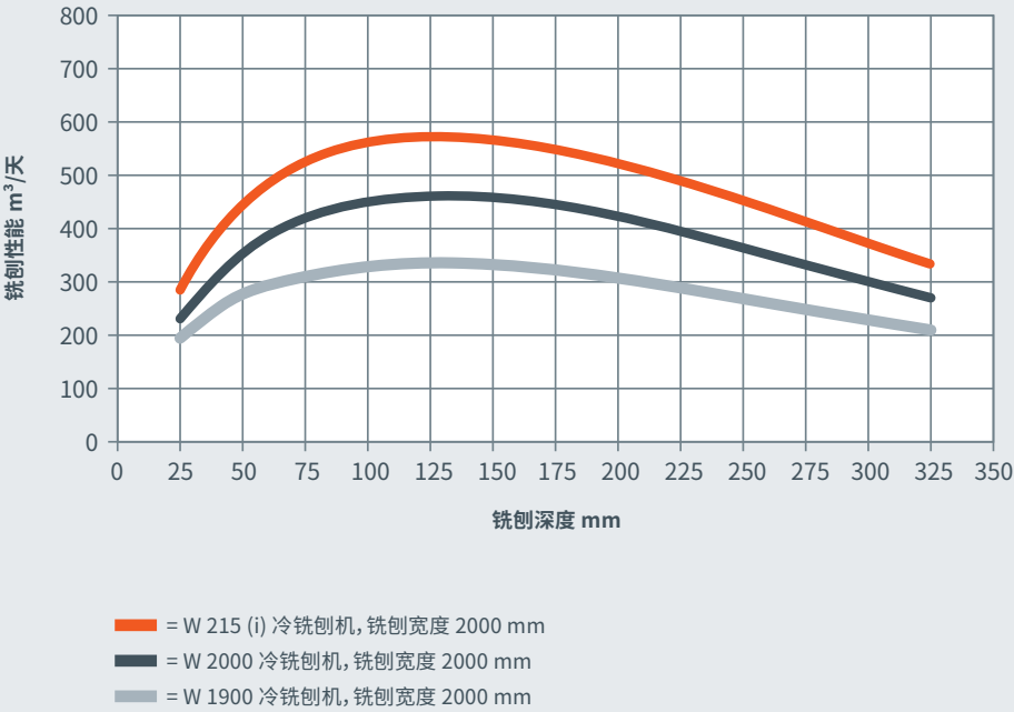
中等硬度沥青的铣刨性能
