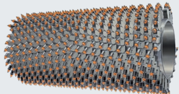
精铣刨转子，刀间距 6x2 mm
