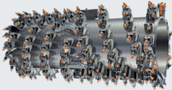
标准型铣刨转子，刀间距 18 mm
