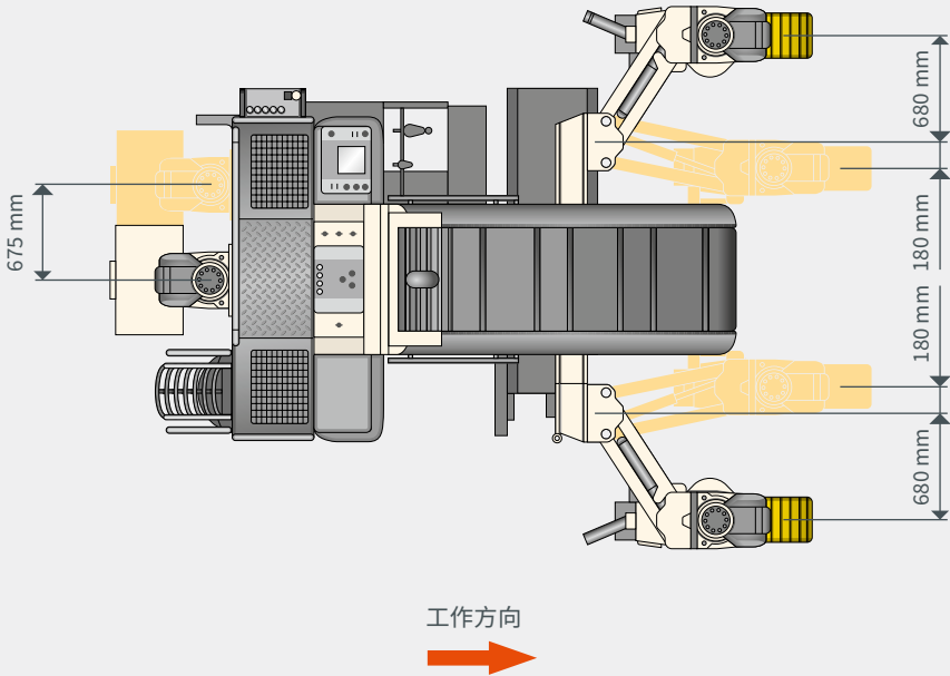
履带配置和附加配置
