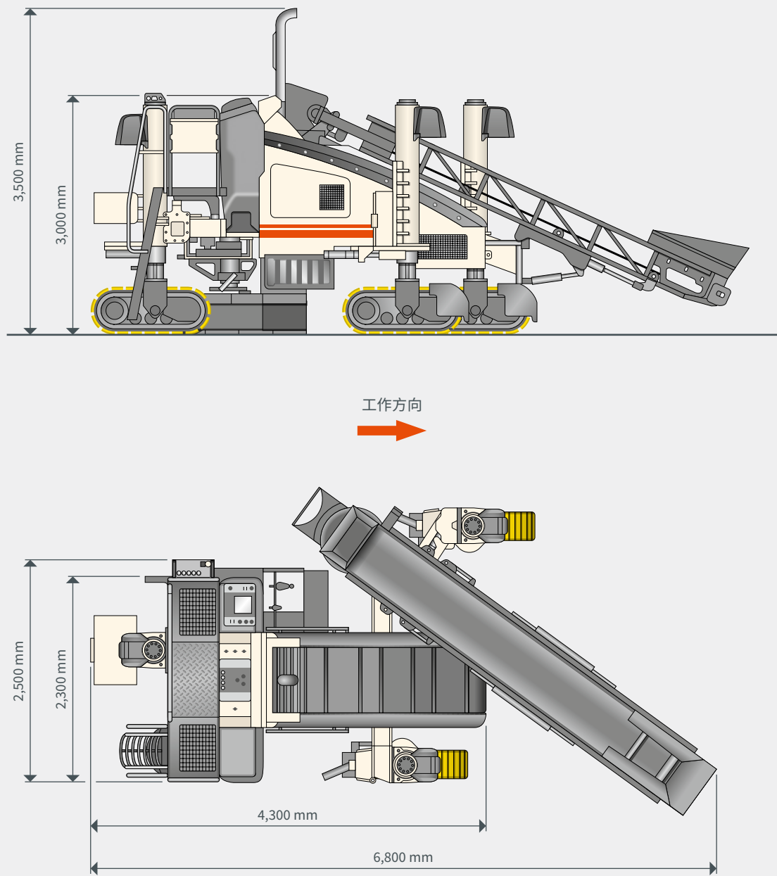
SP 15 (i) 侧视图 / 俯视图
