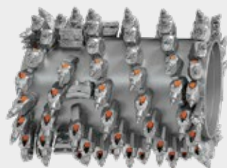
Tambour de fraisage standard Largeur de fraisage : 1 200 mm Profondeur de fraisage : 0 - 330 mm Écartement des pics : 15 mm
