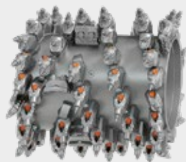
Tambour de fraisage standard Largeur de fraisage : 1 000 mm Profondeur de fraisage : 0 - 330 mm Écartement des pics : 15 mm
