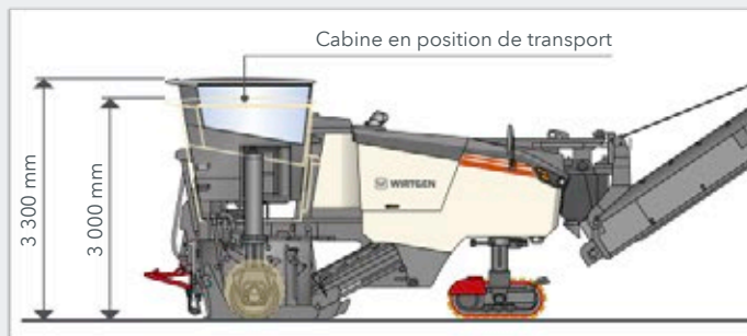
W 100 Fi, W 120 Fi, W 130 Fi avec cabine
