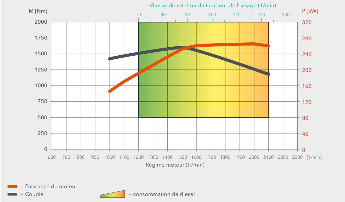
Courbes caractéristiques du moteur des fraiseuses à froid W 100 Fi, W 120 Fi et W 130 Fi
