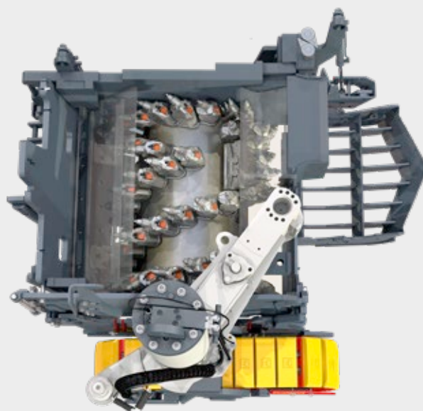
Tren de rodaje en «Posición básica».
