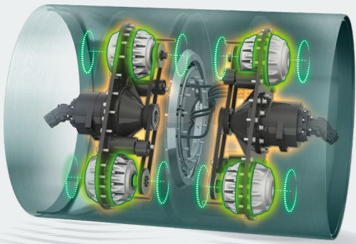
Unique au monde : rouleau divisé avec oscillation.
