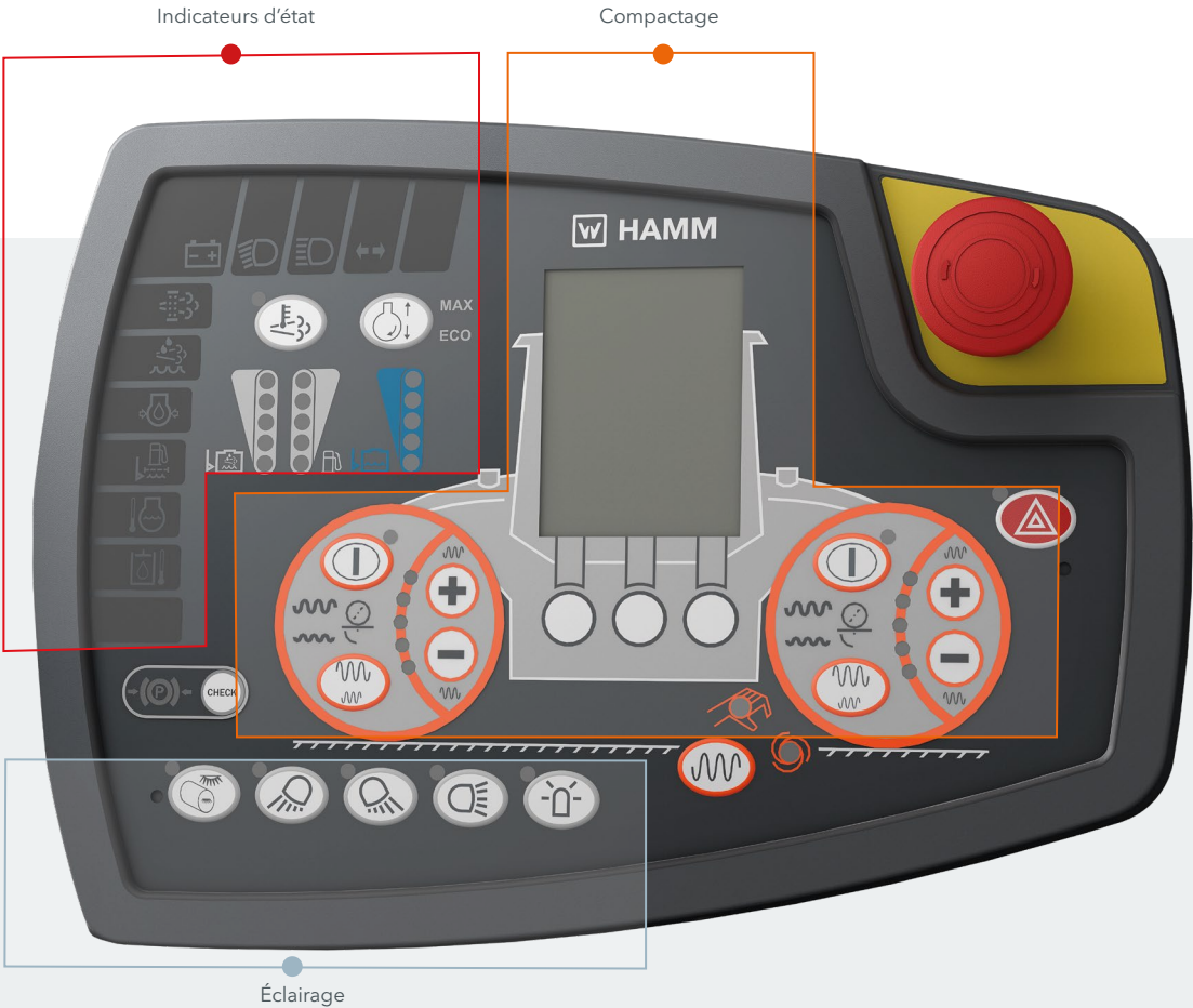
Le tableau de bord près du volant comporte les indicateurs d'état et de paramètres, ainsi que les touches qui sont plus rarement utilisées.
