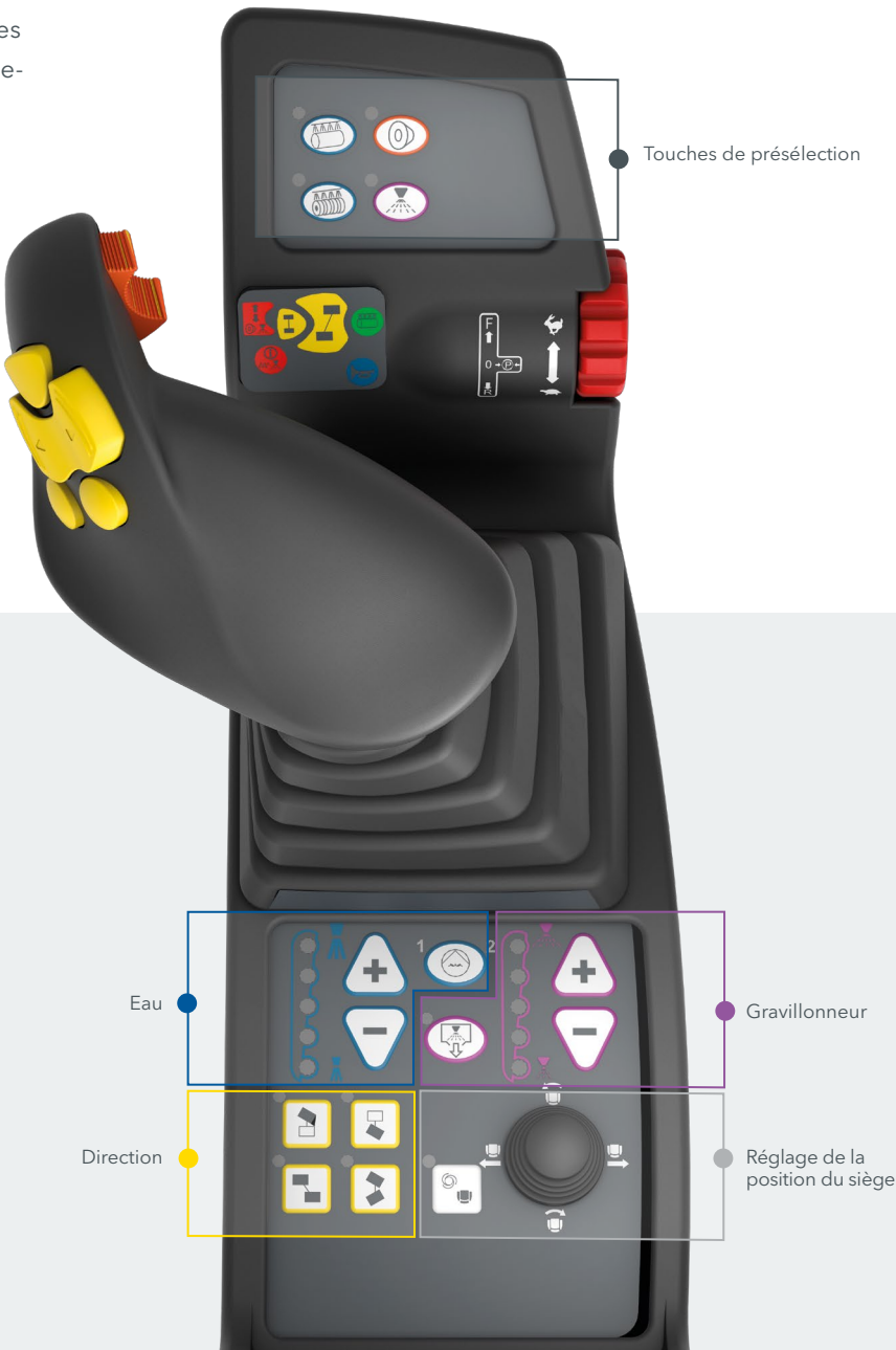
Des conditions claires sur l'accoudoir multifonction : en haut se trouvent les touches de présélection et en bas, les touches de réglage des fonctions.
