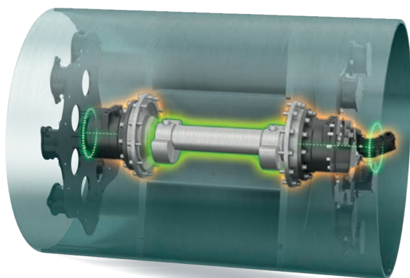
Cylindre vibrant
