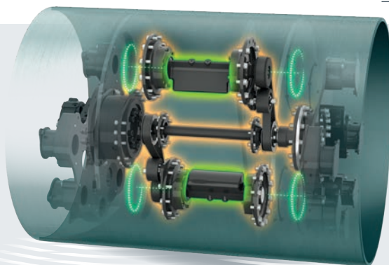
Cylindre oscillant
