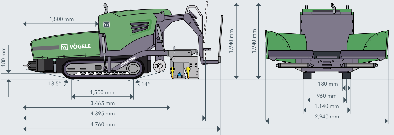
侧视图和前视图
