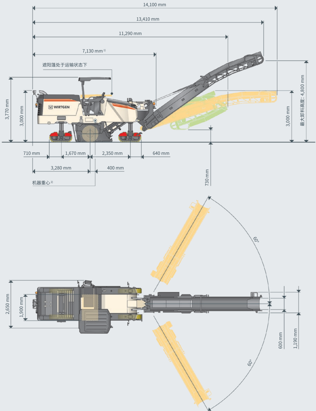
W 185 CF 侧视图 / 俯视图
