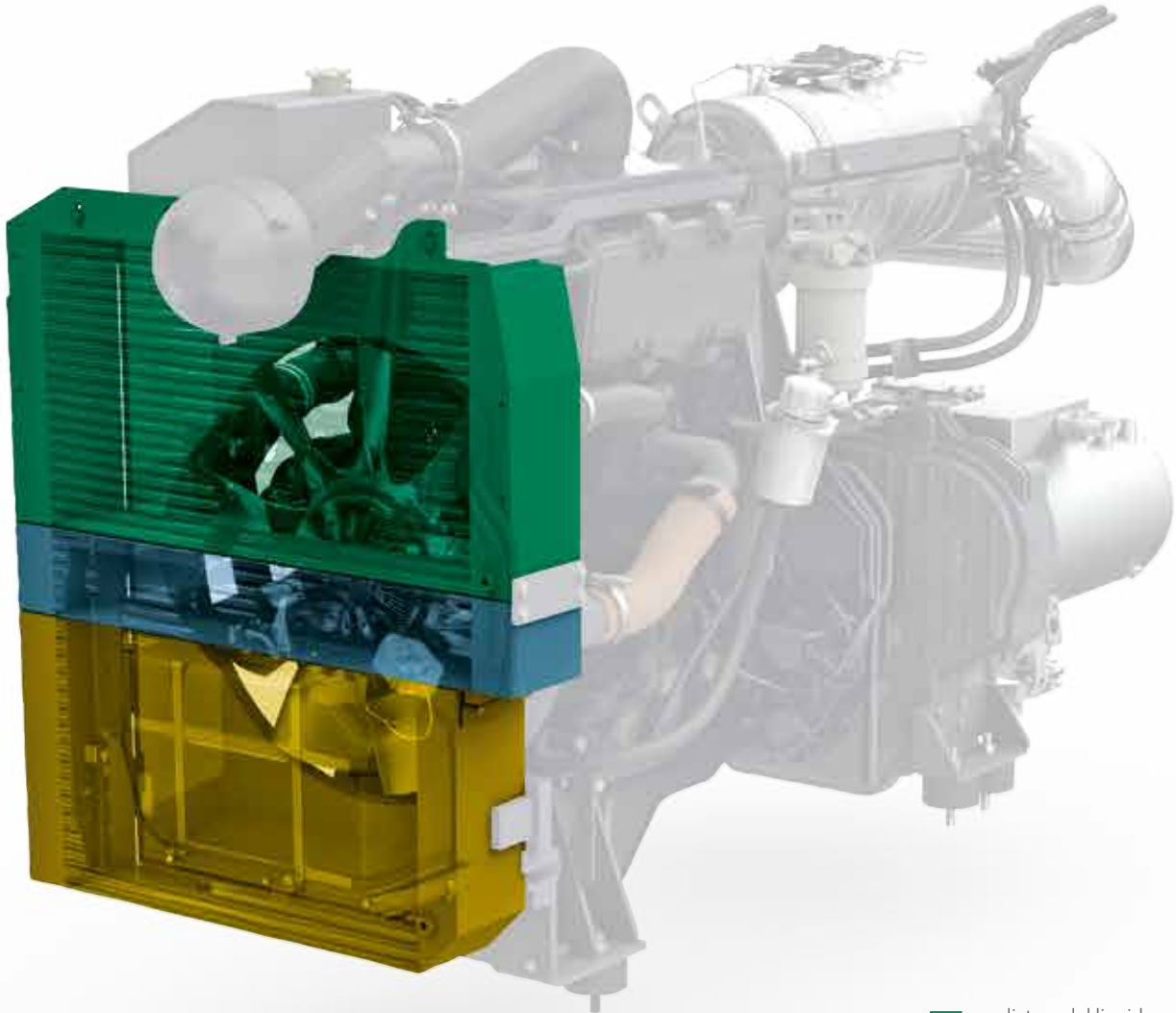
■ = radiatore del liquido refrigerante ■ = intercooler ■ = radiatore dell'olio idraulico
