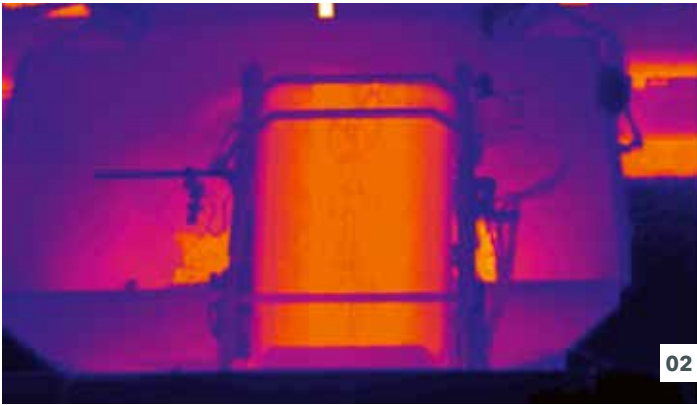
02 Convoieur à bande L'enrobé homogénéisé est acheminé en douceur par le convoieur à bande en forme d'auge jusqu'à la trémie tampon du finisseur.
