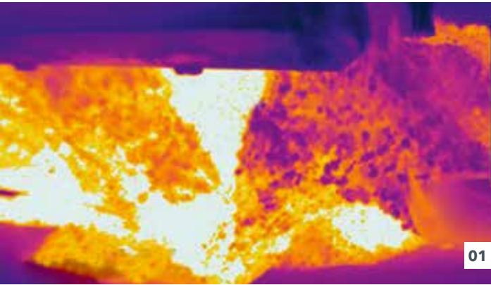
01 Trémie de déversement L'image thermique montre comment les vis coniques transversales homogénéisent l'ensemble de l'enrobé dans la trémie de déversement de l'alimentateur en mélangeant de l'enrobé des zones périphériques plus froides aux zones plus chaudes situées au centre de la trémie.
