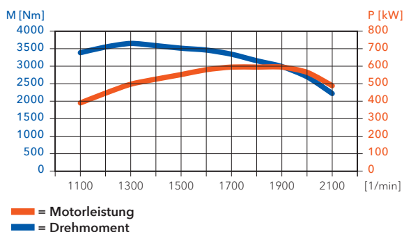
MOTORKENNLINIEN KALTFRÄSE W 220 Fi
