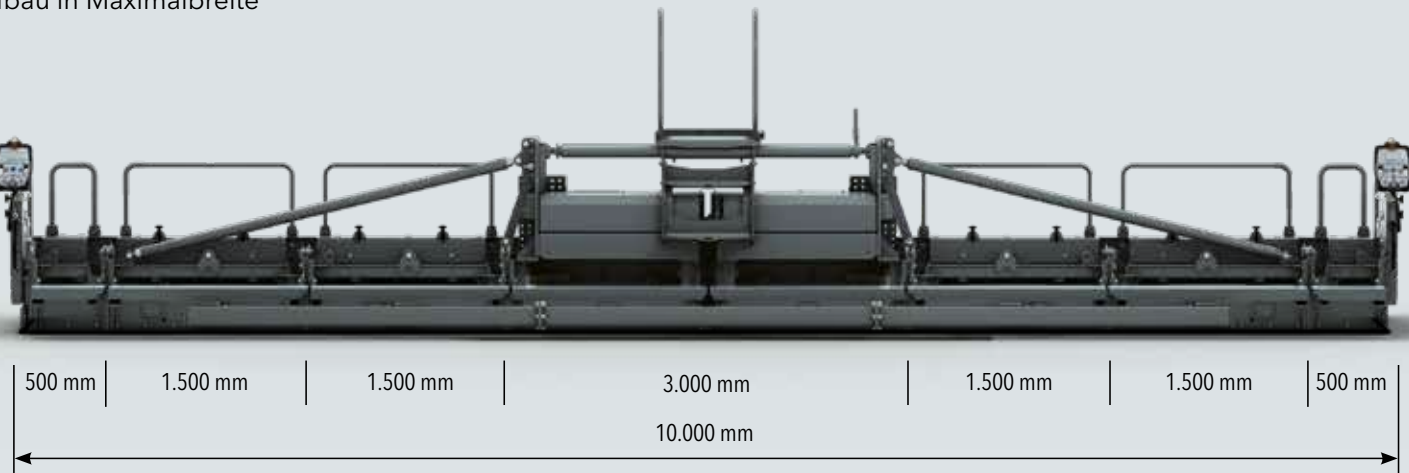
SB 300 HD Aufbau in Maximalbreite
