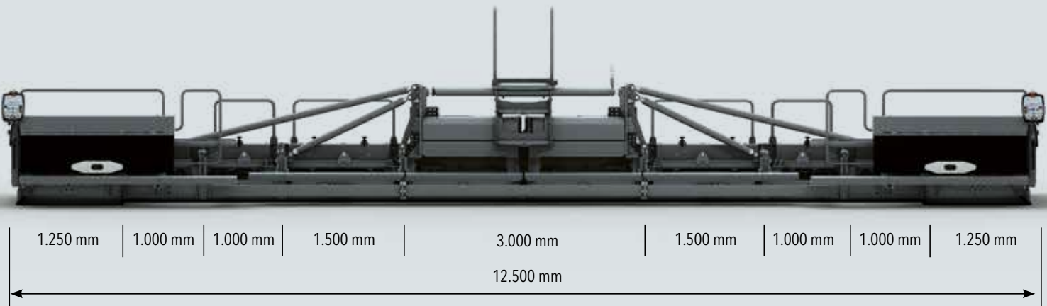
SB 300 TV Aufbau in Maximalbreite
