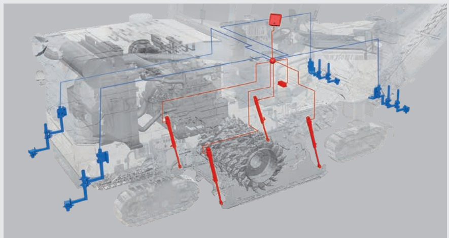
Multiplex-System mit bis zu vier Ultraschallsensoren
