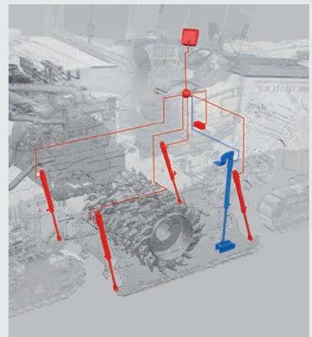
Abtastung vor der Fräswalze
